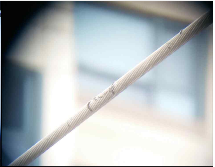
전력선 아크 흔적
