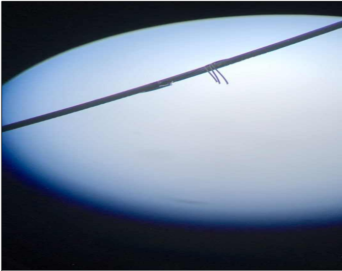
크레인 근접고장으로 인한 전력선 소손
